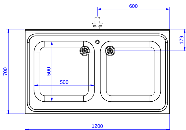
Felülnézet
